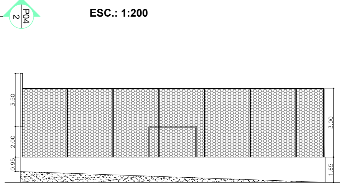
2 - CORTE 2-2 ESC.: 1:200
