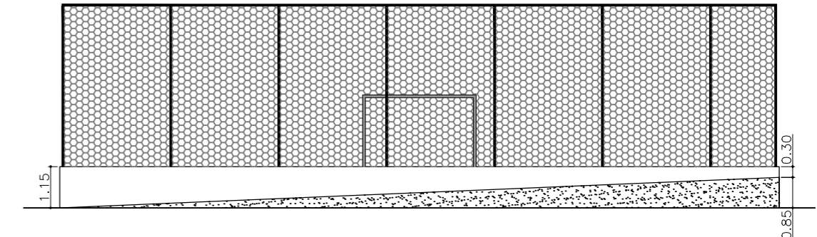
3 - CORTE 4-4 ESC.: 1:200
